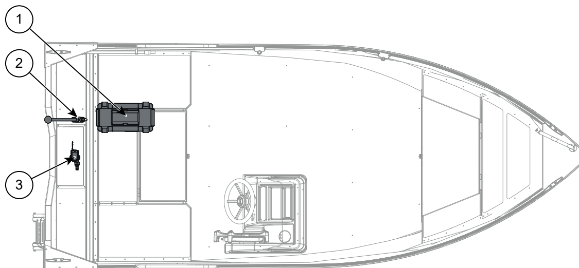
Kuva 8.2 Buster XSr sähkölaitteet
