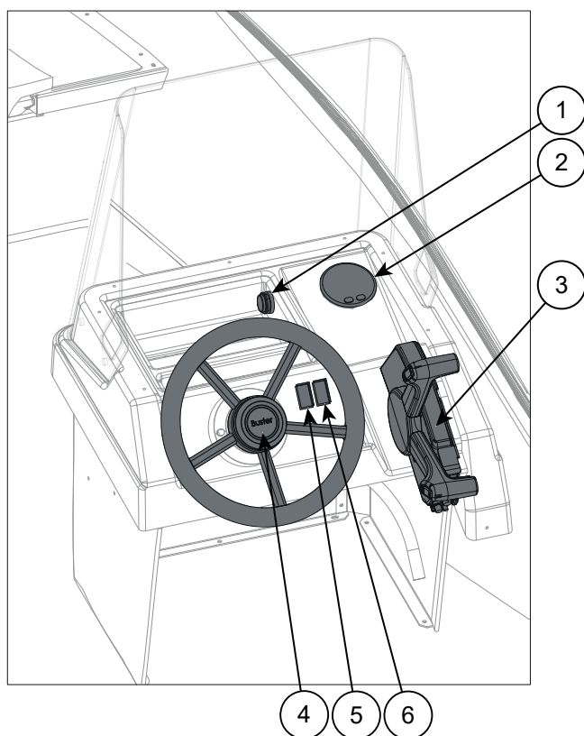
Kuva 5.1 Buster XSr ohjauspisteen hallintalaitteet
