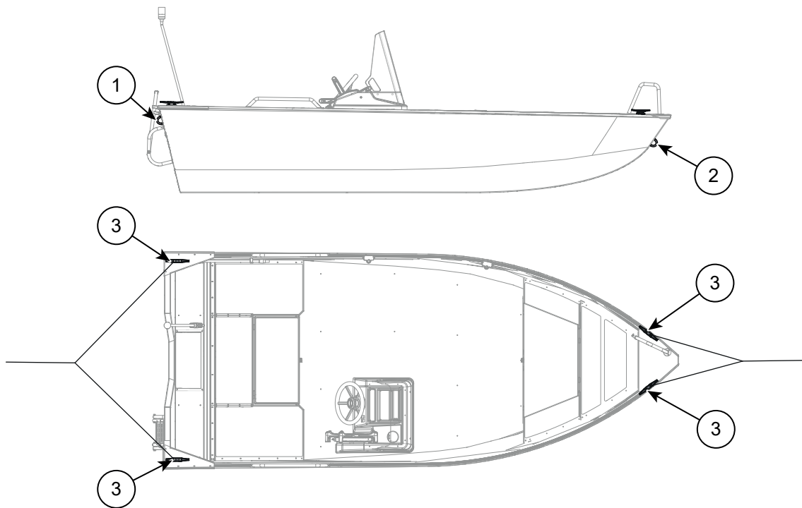
Kuva 5.3 Buster XS/XSr kiinnitys- ja hinauspuisteet
