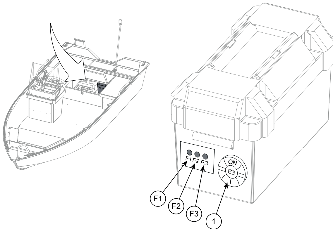
Kuva 8.1 Buster XSr päävirtakytkin ja sulakepaneeli
