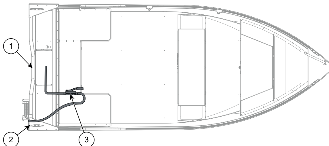
Kuva 9.1 Buster XS tyhjennysvälineet
