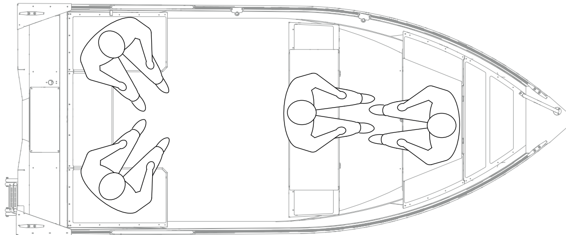
Kuva 4.1 Buster XS istuimet enintään neljälle (4) matkustajalle
